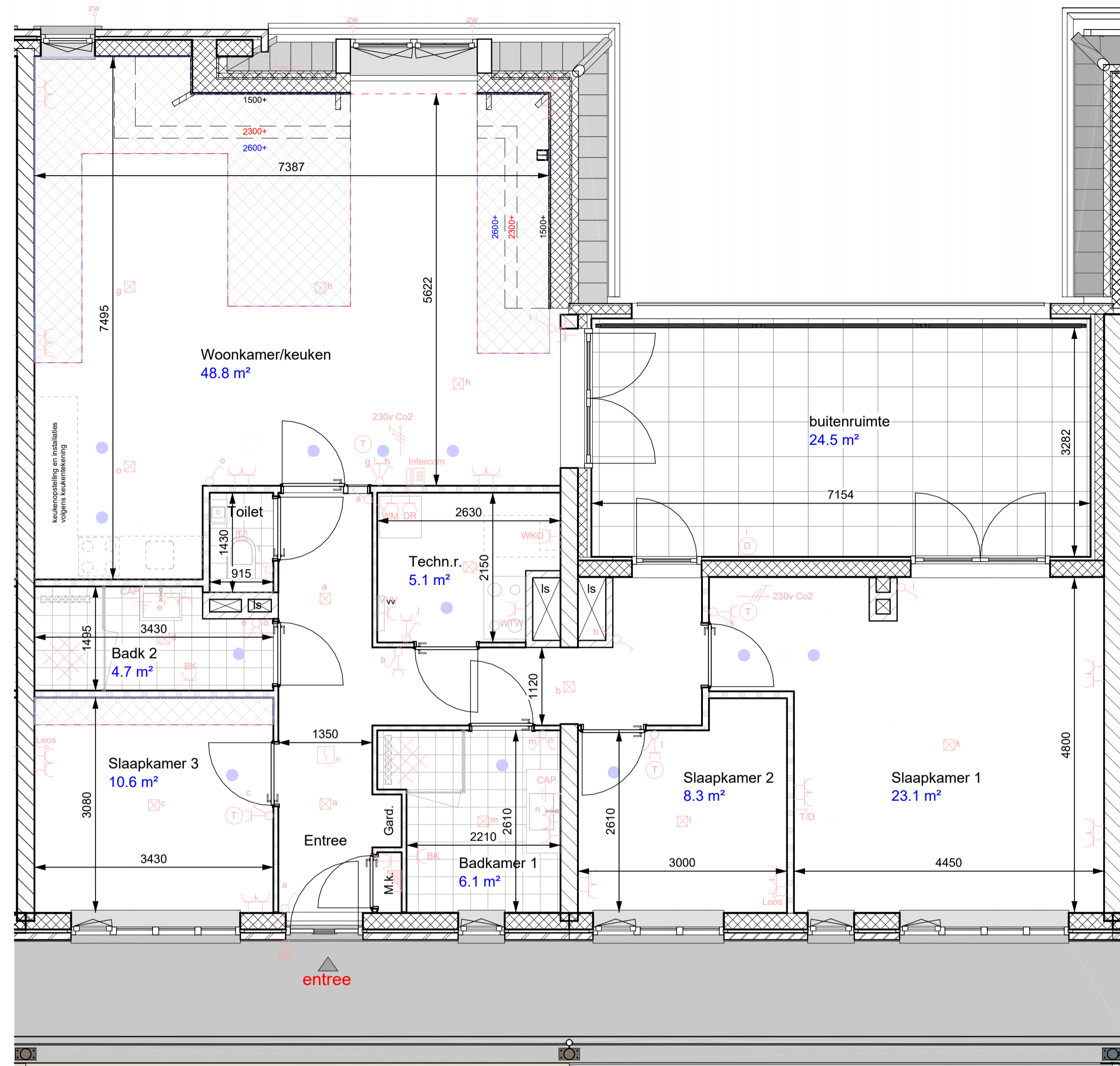
Plattegrond
